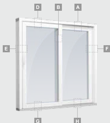
Divdaļīgas paceļamas-bīdāmas durvis Bīdāma vārtne – kreisajā pusē
