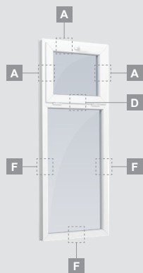
Divdaļīgs logs ar atgāžamu vētrni augšpusē
