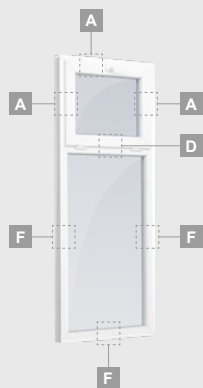
Divdaļīgs logs ar atgāzamu vērtni augšpusē
