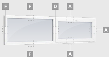
Divdaļīgs logs ar atgāzamu vērtni labajā pusē
